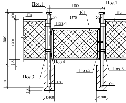
Фрагмент установки калитки К1
