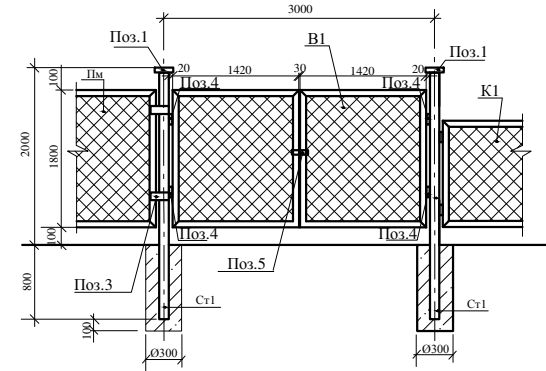
Фрагмент установки ворот В1
