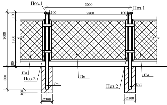
Фрагмент ограждения территории
