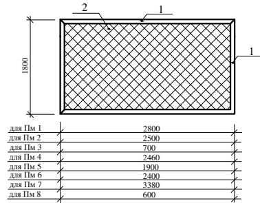
Панели ограждения Пм1:- Пм8.
